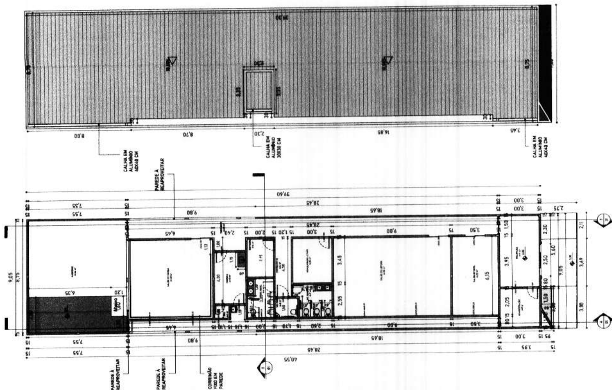
1 TÉRREO 1:100
